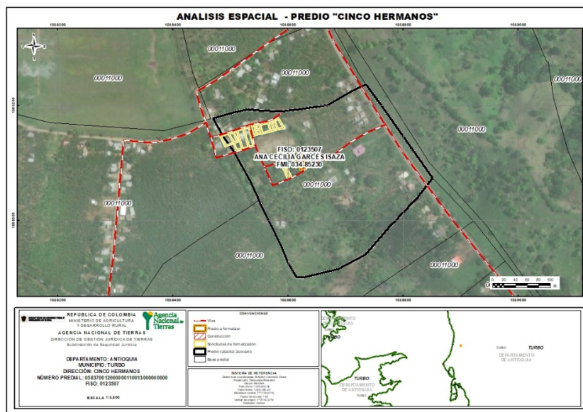
IMAGEN 1 – ANALISIS ESPACIAL
